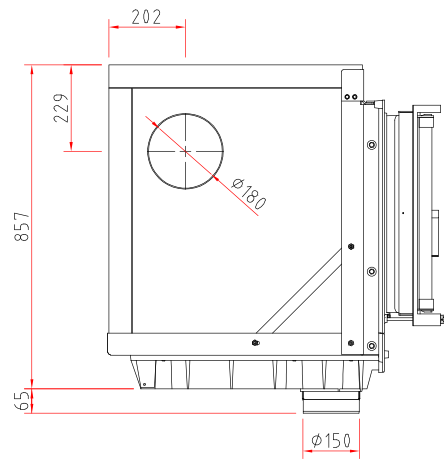
Seitenansicht M 1:20
